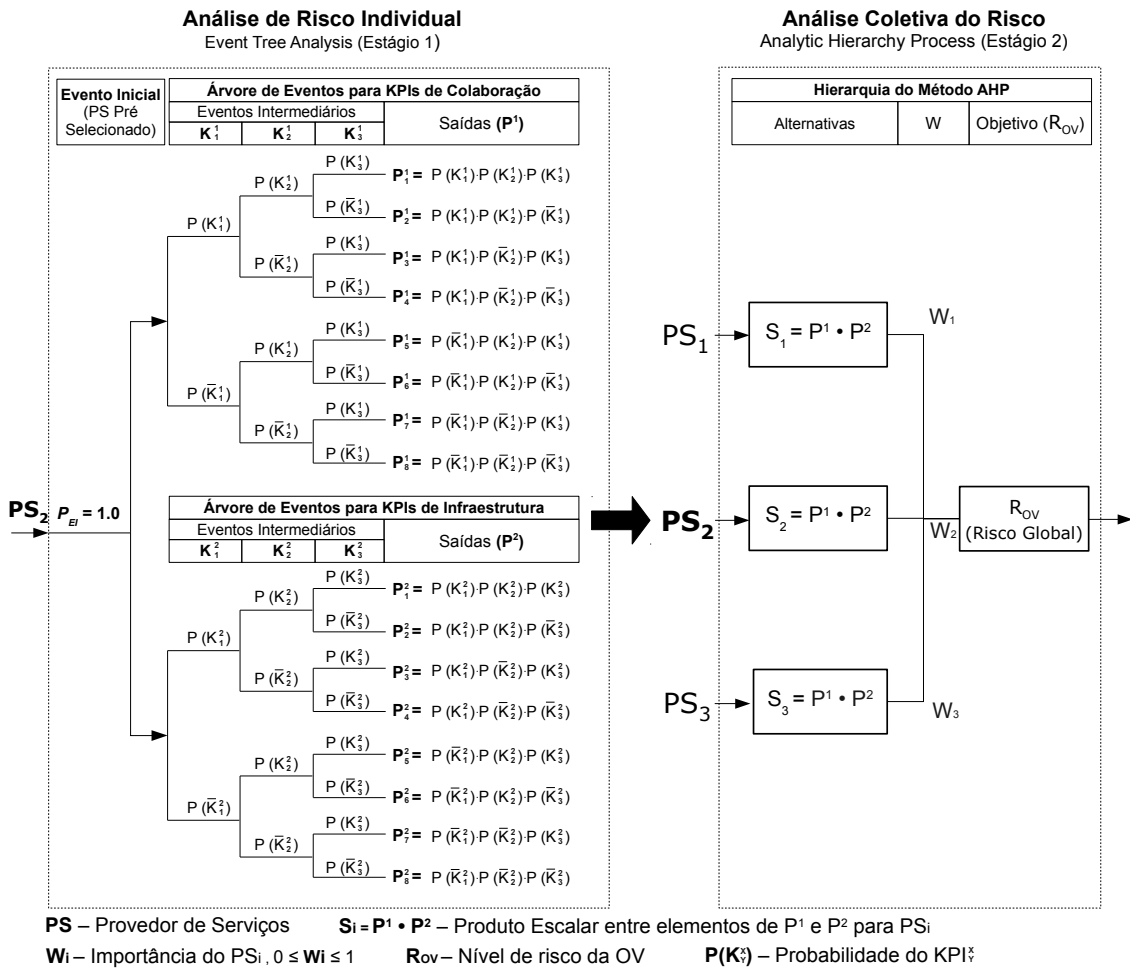
Figura 2. Visão geral do método MAR-SP.
