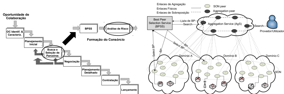
(a) Etapas para a criação de uma OV. Adaptado de [Camarinha-Matos and Afsarmanesh 2005]
