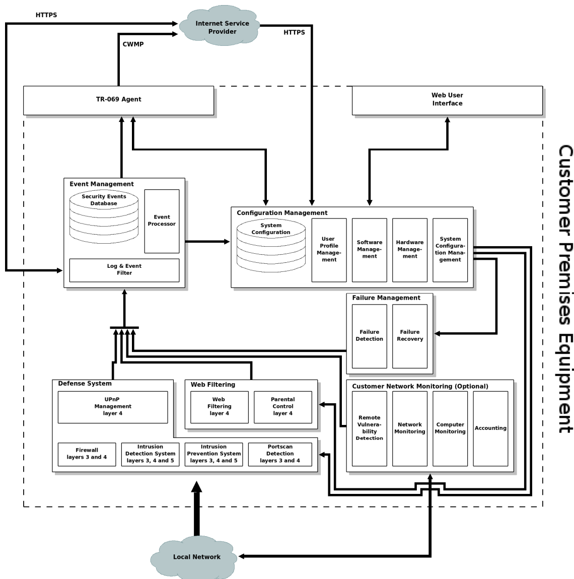
Figura 5. Arquitetura da Plataforma S3P (CPE)
